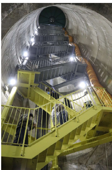
→ 立坑内部
